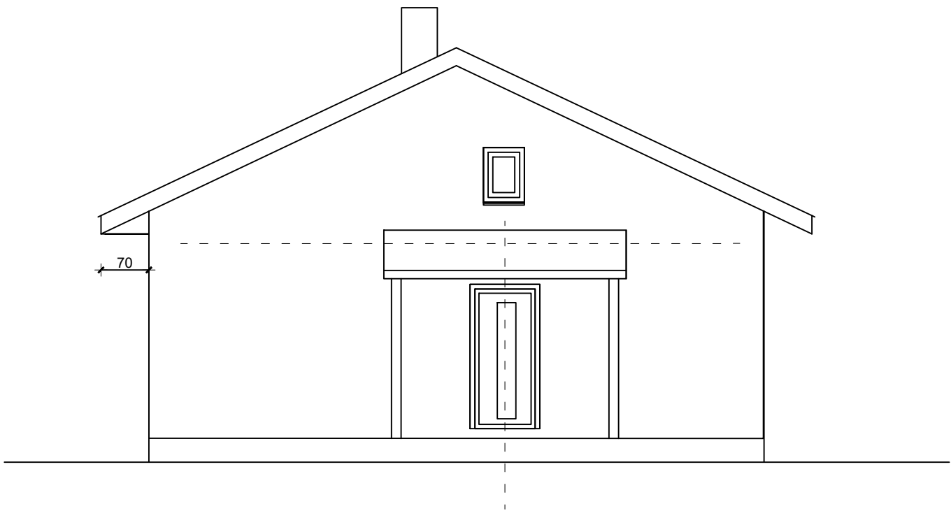
SJEVER mj 1:100
