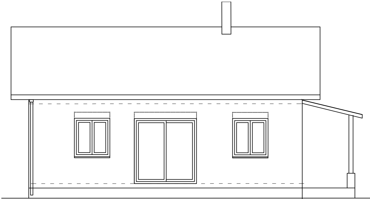
SJEVER mj 1:100
